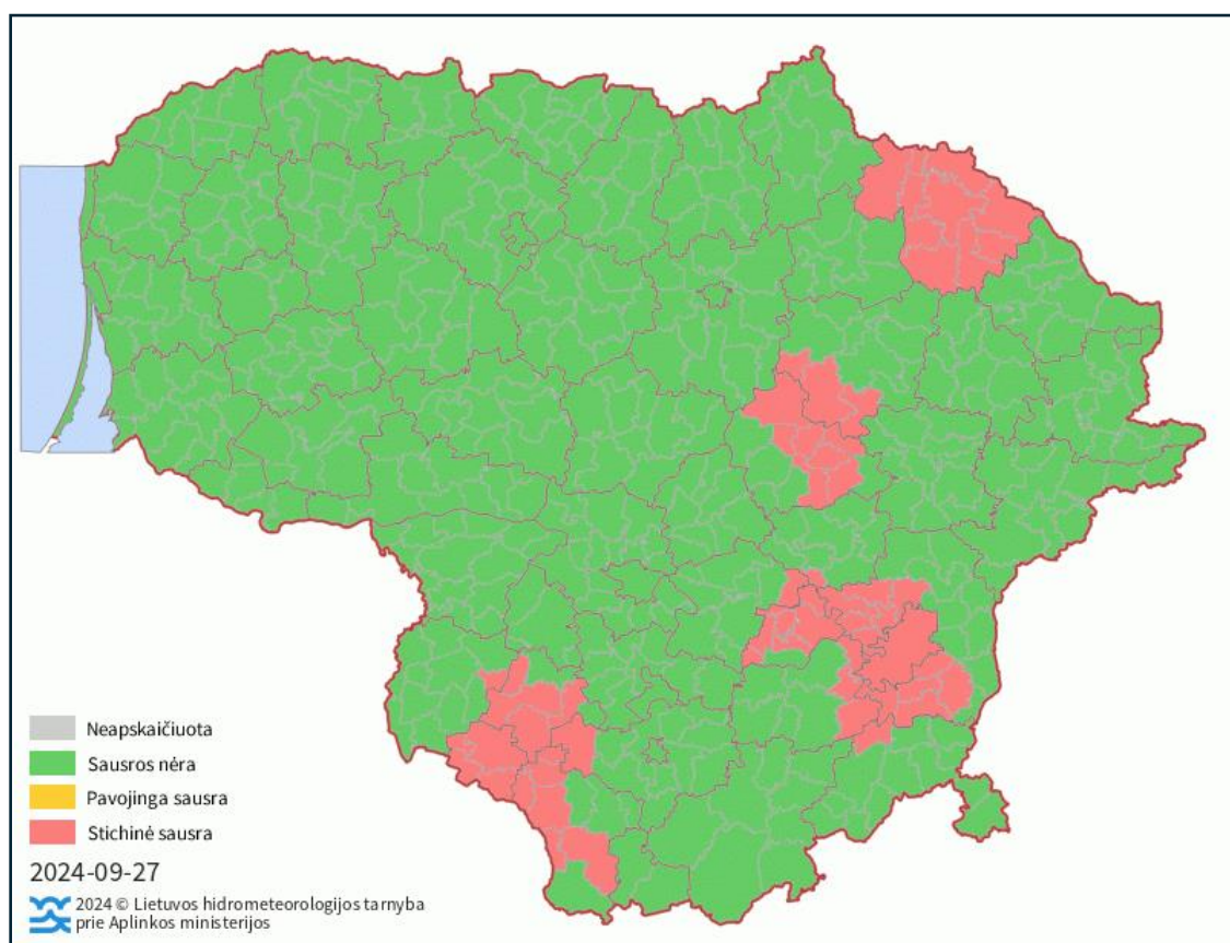
1 pav. Sausros išplitimas savivaldybių teritorijose 2024-09-27
