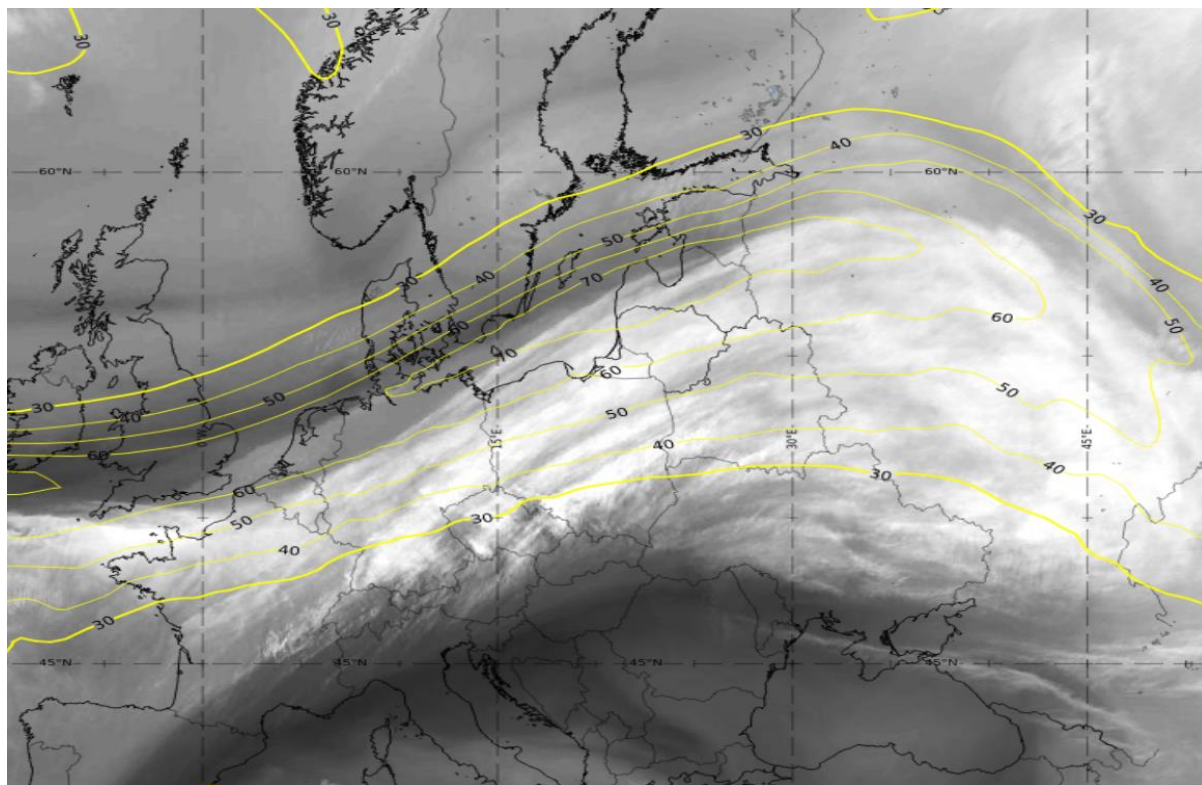
MSG palydovo vandens garų kanalo vaizdas su stipriausių vėjų sritimi (m/s, geltonos izolinijos) 7 km aukštyje (sausio 2 d. 2 val.)
